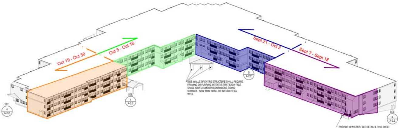
7 NE ISOMETRIC
